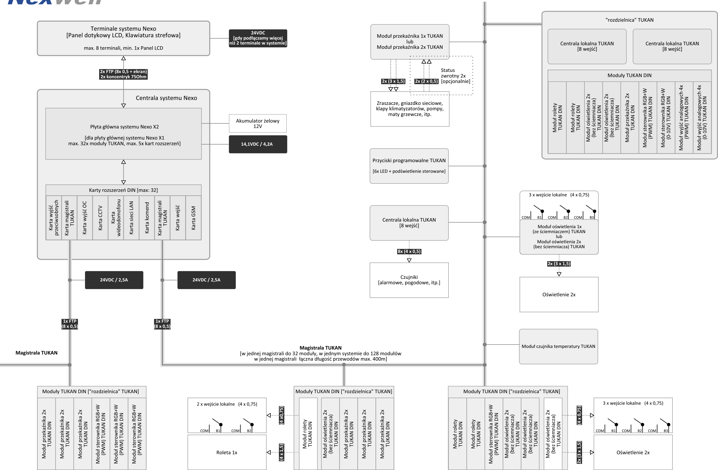
Struktura systemu Nexu - magistrala TUKAN
